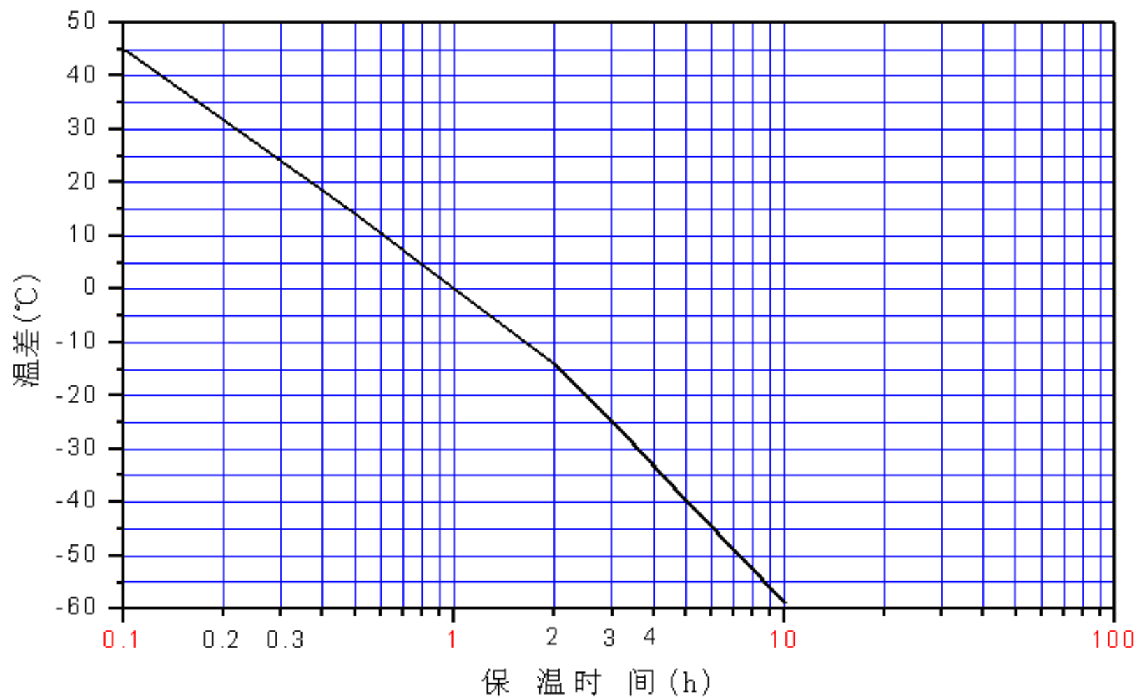
BQS 温度校正曲线 (900℃ -1200℃)
